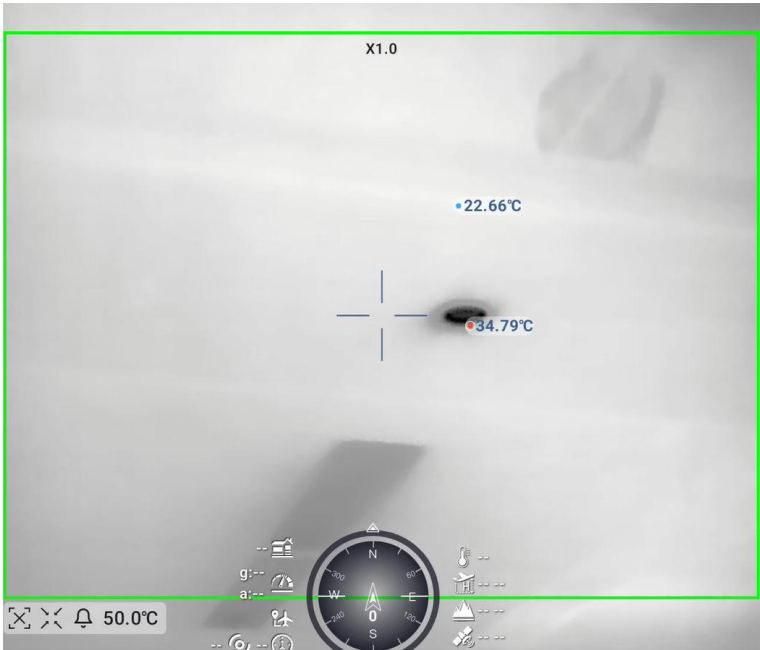
黑热
