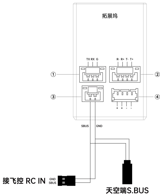
接线示意图
